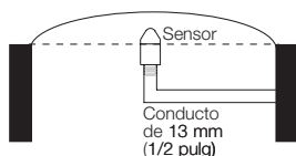
Montaje del GRX-CESI: Montaje en pared de reflexión
