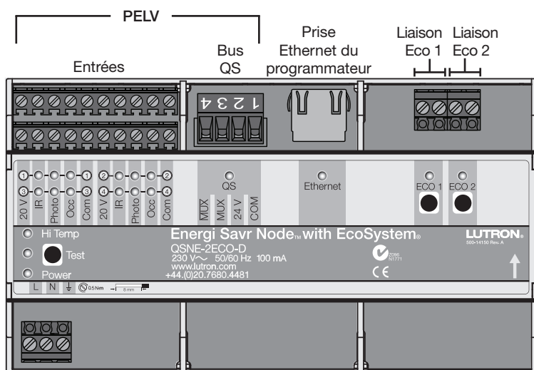
Câblage du secteur
