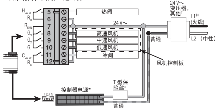
接线图 2 (风机盘管机组)
