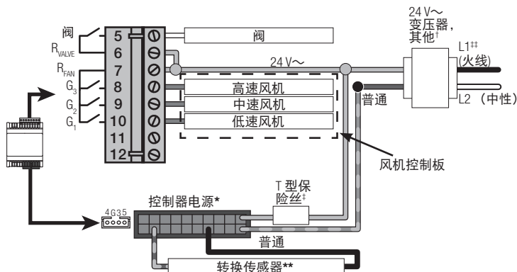
接线图 2 (风机盘管机组)
