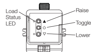
PowPak Wireless Fixture Control (FCJS-010/FCJS-010-EM or FCJS-ECO/FCJS-ECO-EM)
