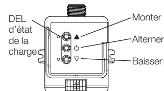
Commande de luminaire sans fil PowPak (FCJS-010/FCJS-010-EM ou FCJS-ECO/FCJS-ECO-EM)
