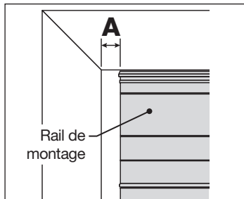
Dégagement minimum « A » Store avec façade : 6 mm (1/4 po)
