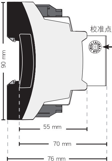
侧视图
