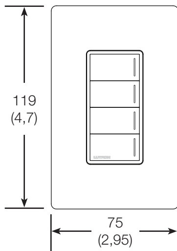
Vue frontale
