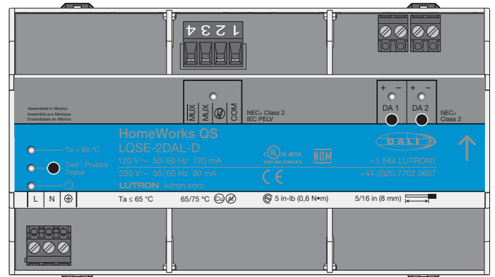
DALI®-Leistungsmodul (LQSE-2DAL-D)
