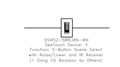
QSW2-5BRLIRN
