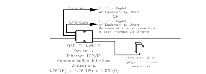
QSE-CI-NWK-E & T120-15DC-9-BL
