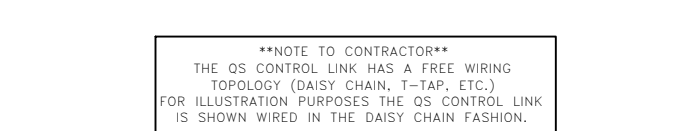
WIRING NOTE-DAISY CHAIN-QS
