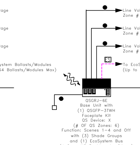
QSGRJ-6E + 3 Shades
