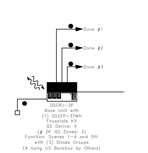
QSGRJ-3P + 3 Shades
