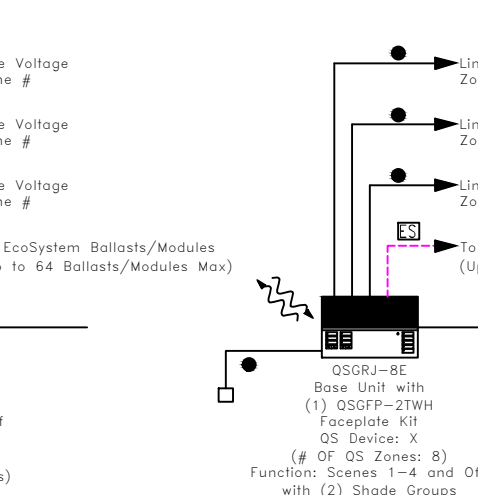
QSGRJ-8E + 2 Shades
