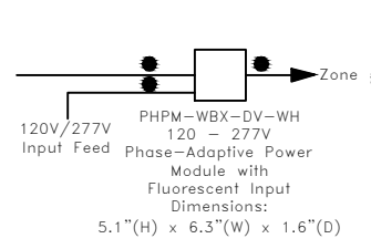
PHPM-WBX-DV-WH
