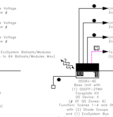
QSGRJ-6E + 2 Shades
