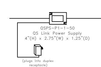
QSPS-P1-1-50
