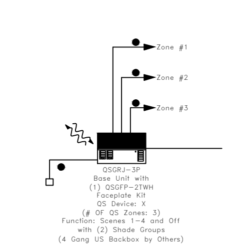
QSGRJ-3P + 2 Shades
